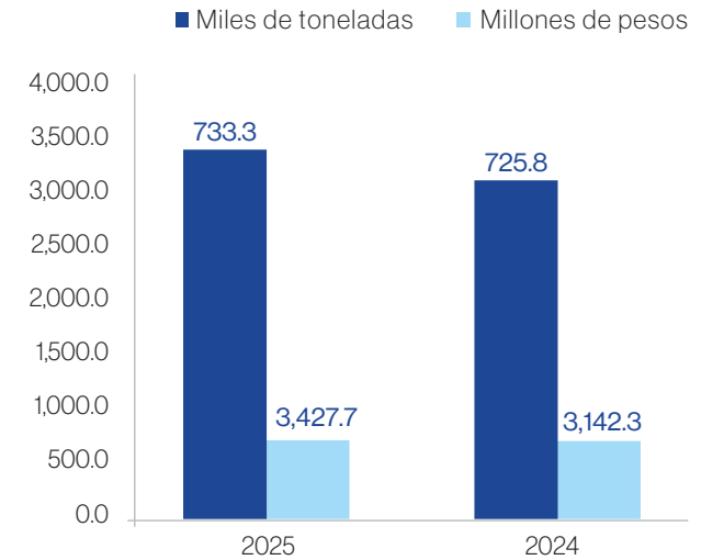
VOLUMEN Y VALOR DE LA PRODUCCIÓN DE SULFATO DE SODIO
